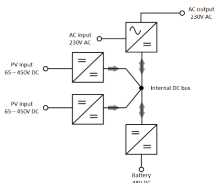
Blockdiagramm von Multi RS Solar
