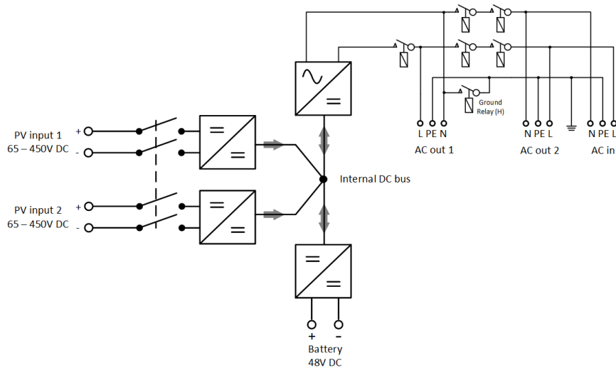
Abbildung 4. Multi RS Solar
