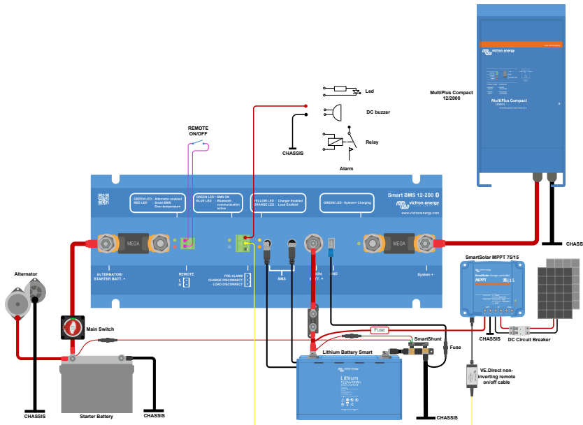
Anwendungsbeispiel mit MultiPlus Compact und MPPT
