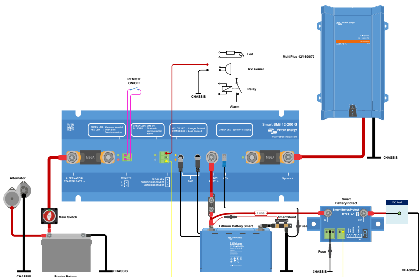
Anwendungsbeispiel mit MultiPlus und Smart BatteryProtect
