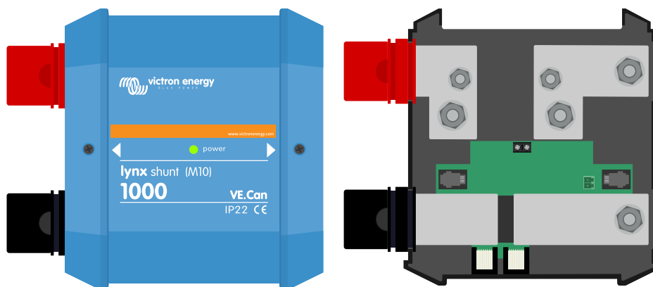
Der Lynx Shunt VE.Can (M8) – mit und ohne Schutzabdeckung
