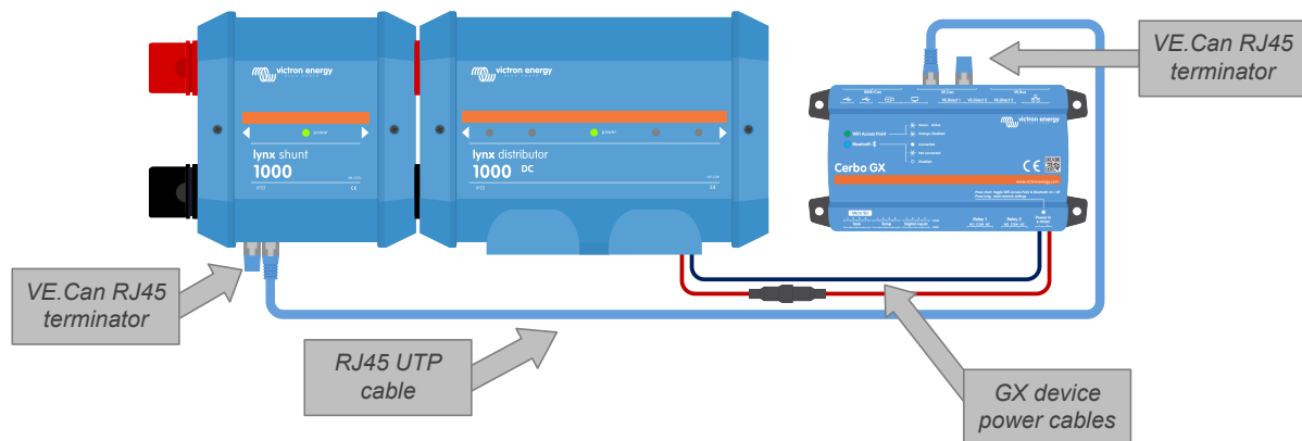
Verkabelungsbeispiel Lynx Shunt VE.Can und GX-Gerät
