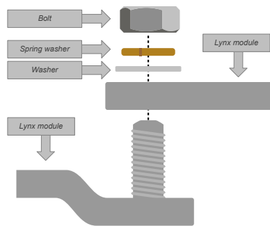
Abbildung 3. Anschlussreihenfolge beim Anschluss von zwei Lynx-Modulen
