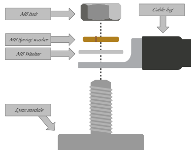
Abbildung 4. Richtige Montagesequenz der Gleichstromleitungen
