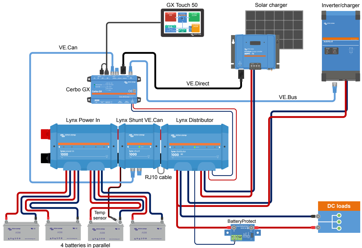
System mit Lynx Shunt VE.Can, Blei-Säure-Batterien und einem Lynx Distributor
