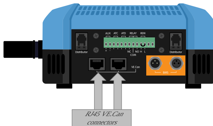
Position der VE.Can-Steckverbindungen auf dem Lynx Smart BMS NG
