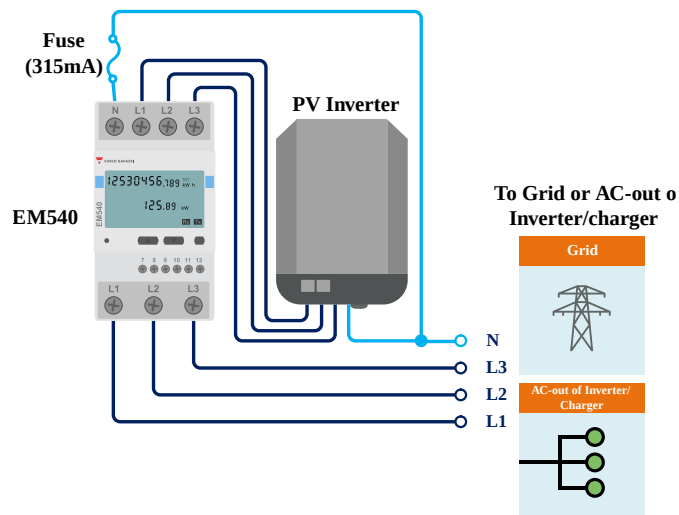
EM540 verkabelt zur Messung eines 3-Phasen-Wechselrichters – beachten Sie, dass die Klemmen 1, 2 und 3 dem PV-Wechselrichter zugewandt sind
