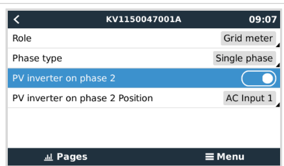
Einphasig mit Doppelfunktion zur Messung des Netzes auf L1 und eines PV-Wechselrichters auf L2. Bitte beachten Sie, dass dies nur für den EM540 und ET340 gilt.
